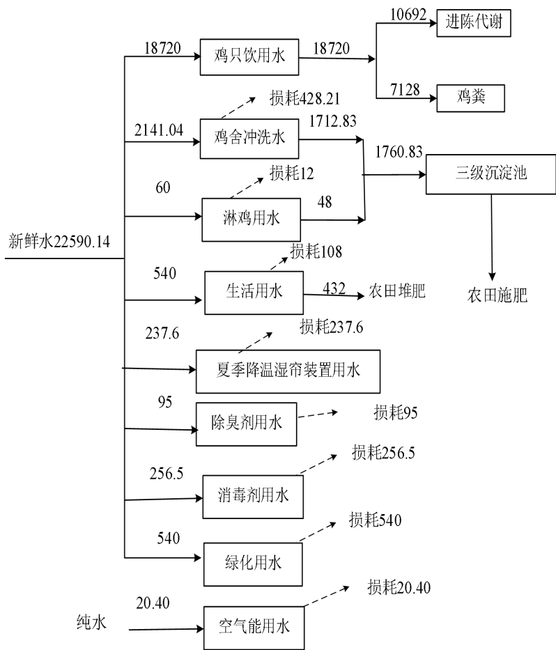
图 3.4-1 项目水平衡图(m³/a)
